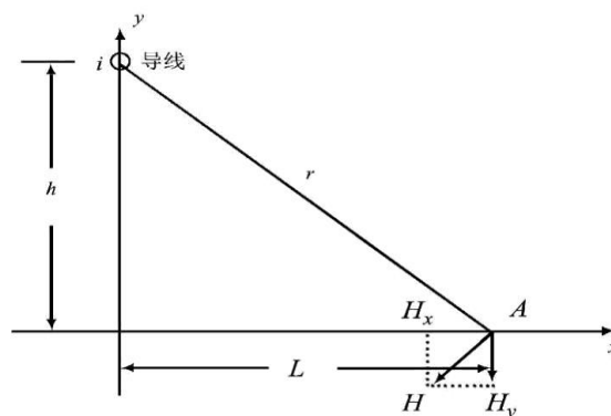
图 3.1-4 磁场向量图
