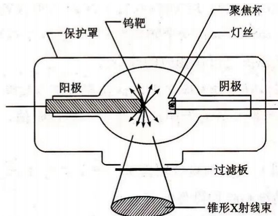
图 9-1 典型的 X 射线管结构图
