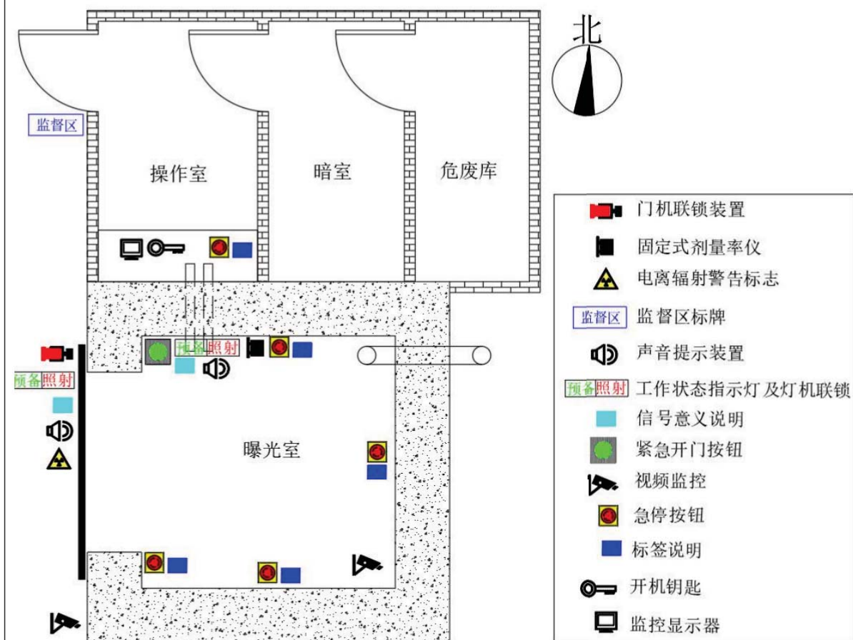
图 10-2 本项目辐射安全与防护措施分布图
