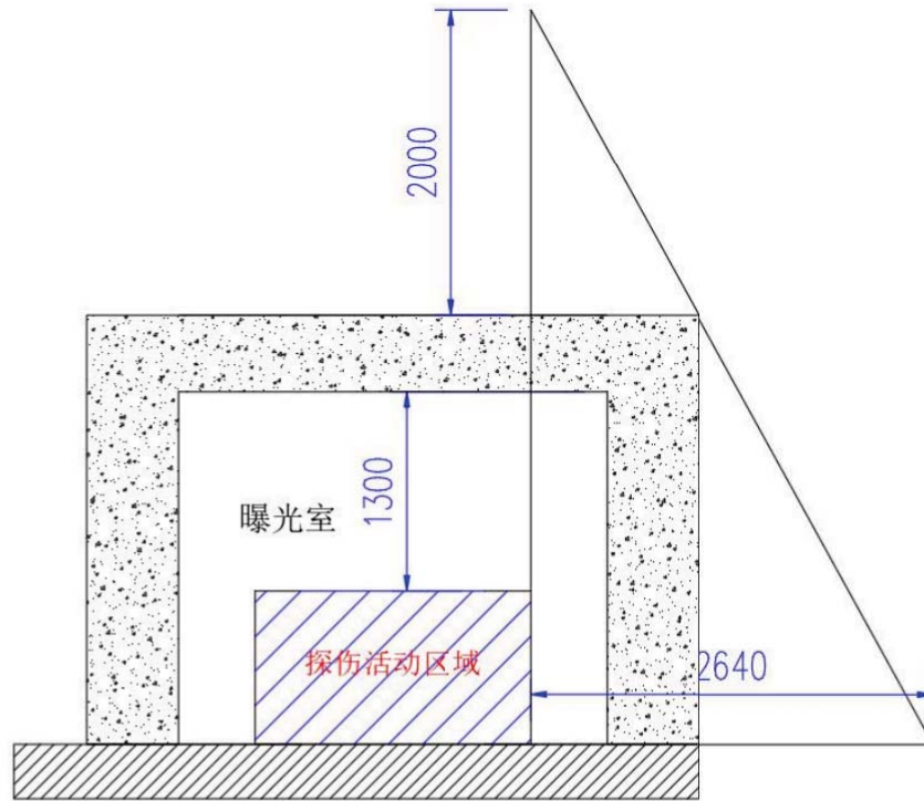
图 11-3 天空反散射示意图
