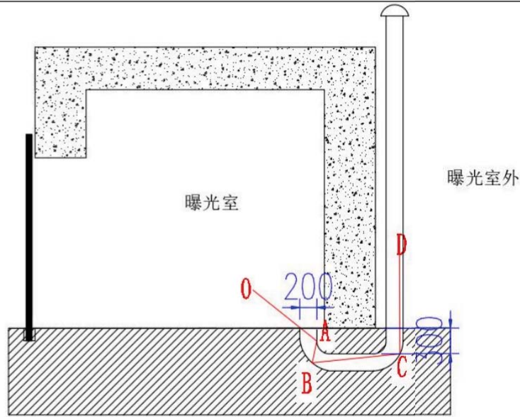
图 11-4 本项目通风管道散射示意图
