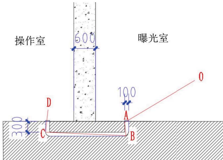
图 11-5 本项目电缆管道散射示意图
