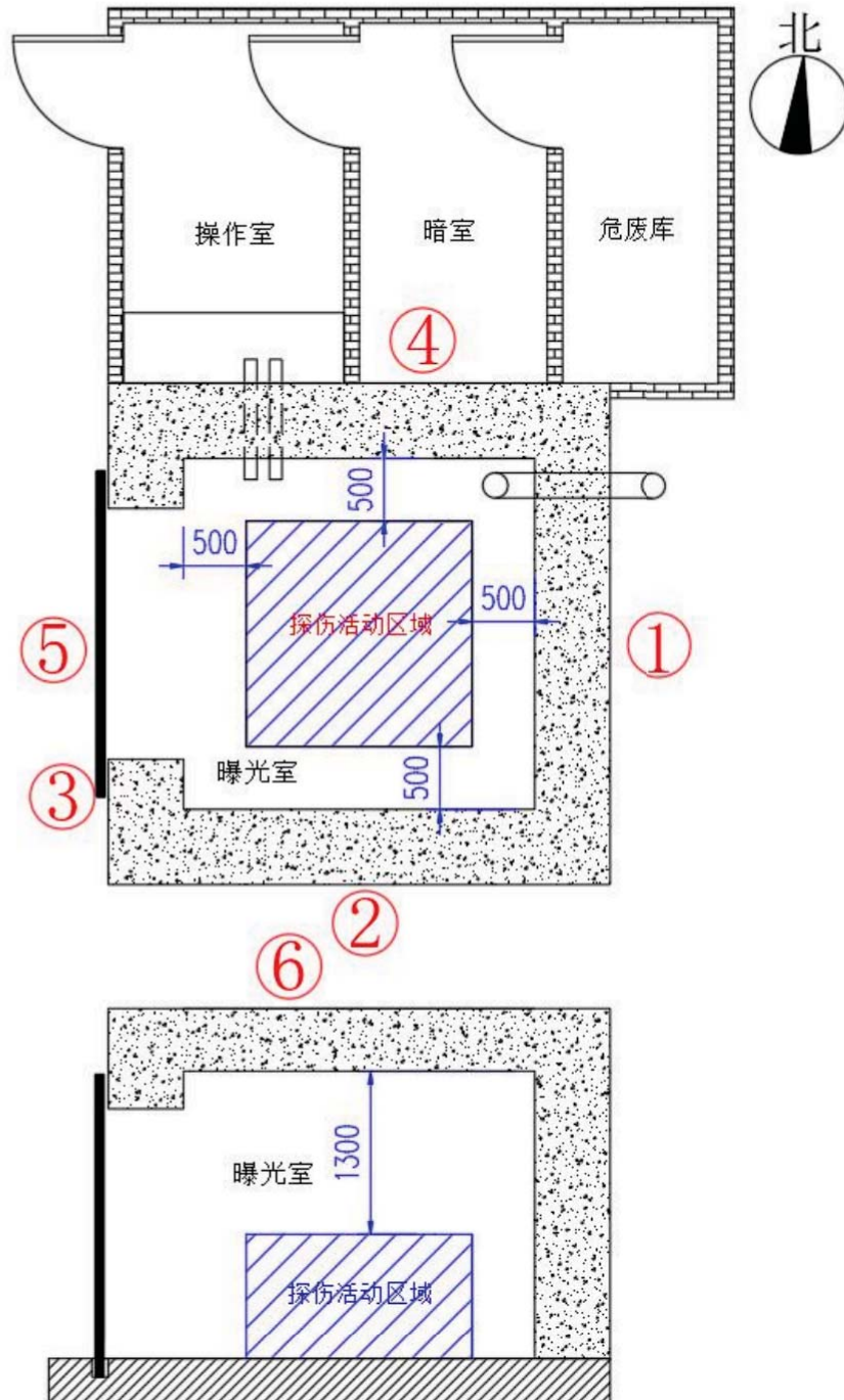
图 11-2 本项目探伤房计算点位示意图 (单位: mm)
